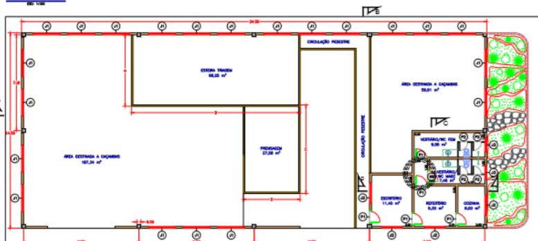
PLANTA DO TERREO
