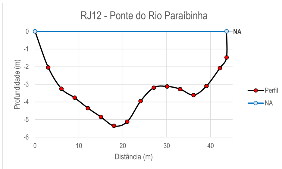
Figura 4.25. Perfil batimétrico da seção de medição do ponto RJ12 - Ponte Rio Paraibinha.
