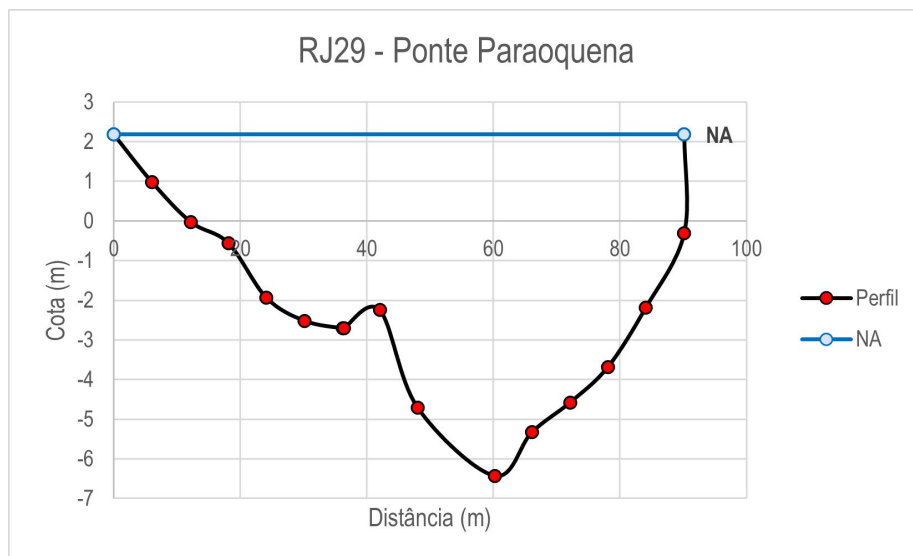
Figura 4.59. Perfil batimétrico da seção de medição do ponto RJ29 - Ponte Paraquena.
