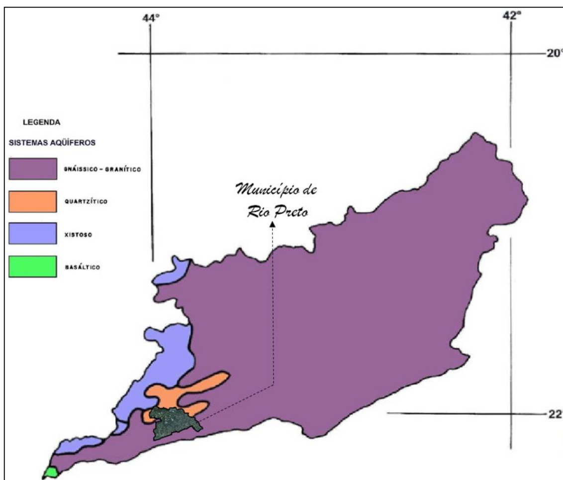
Figura 22 - Sistemas aquíferos existentes no trecho mineiro da Bacia do Rio Paraíba do Sul e a localização do município de Rio Preto no aquífero gnásico-granítico e quartzítico
