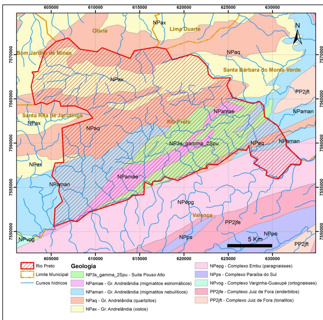
Figura 18 - Mapa geológico da região de Rio Preto
